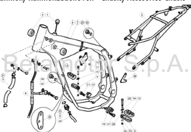
TAV.31-32 Telaio/Accessori telaio - Frame/Frane accessories - Chassis/Accessoires chassis - Rahmen/Rahmenzubehör en - Chasis/Accesorios Chasis
