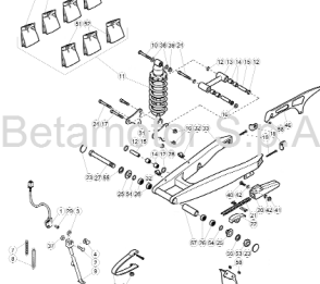
TAV.33 Sospensione posteriore/Forcellone - Rear suspension/Rear fork - Suspension arrière/Fouche arrière - Hinterfederung/Hinterradschwinge - Suspensión trasera/Horquilla posterior
