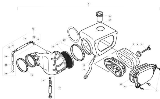
TAV.38 Scatola filtro - Filter box - Boî tier du filtre - Sicherungskasten - Caja del filtro
