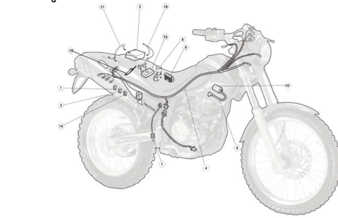
TAV.40A Impianto elettrico - Electrical equipment - Installation electrique - Elektrische anlage - Instalació n electrica
