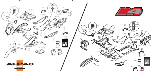
TAV.43 Carenature-Serbatoio-Sella - Fairings-Tank-Saddle - Carenages-Reservoir-Selle - Verkleidungen-Tank-Sattel - Carenados-Deposito-Sillí n
