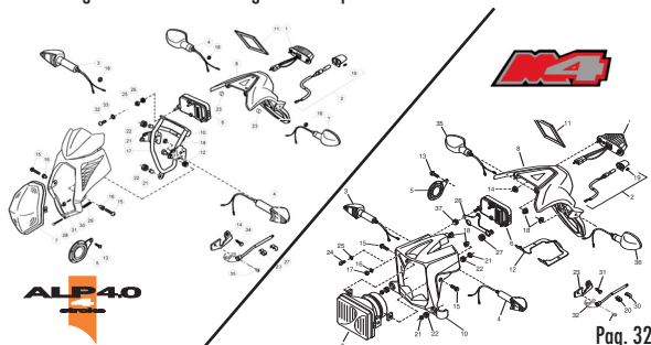
TAV.40 - Fanaleria-dispositivi elettrici - Lights-electric devices - Feux-Dispositifs electriques - Beleuchtung-Elektrische Ausrüstung - Faros-Dispositivos electricos
