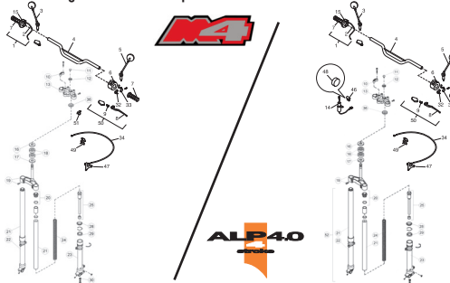
TAV.34 Forcella anteriore-Manubrio - Front fork-Handlebar - Fourche AV-Guidon - Vorderradgabel-Lenker - Horquilla delantera-Manillar
