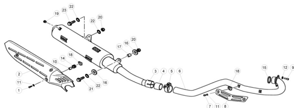
TAV.37 Gruppo scarico - Exhaust system - Echappement - Auspuffanlage - Grupo escape
