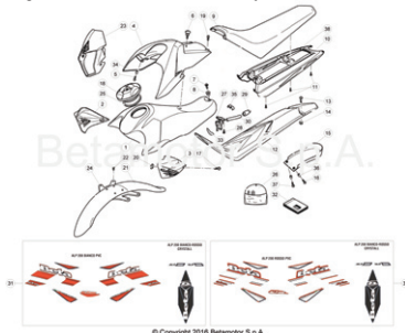
TAV.43 Carenature-Serbatoio-Sella - Fairings-Tank-Saddle - Carenages-Reservoir-Selle - Verkleidungen-Tank-Sattel - Carenados-Deposito-Sillin
