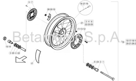
TAV.42 Ruota posteriore - Rear wheel - Roue AR. - Hinterrad - Rueda trasera
