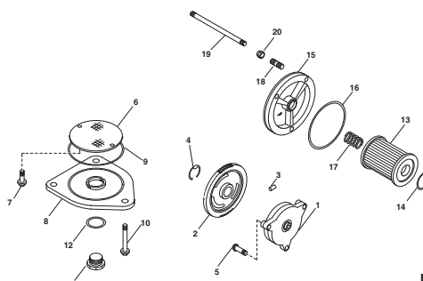
TAV.08 Pompa olio - Oil pump - Pompe d'huile - Ölpumpe - Bomba de aceite
