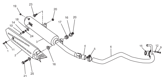
TAV.37 Gruppo scarico - Exhaust system - Echappement - Auspuffanlage - Grupo escape
