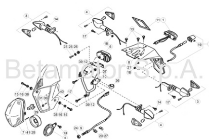
TAV.40B Impianto elettrico - Electrical equipment - Installation électrique - Elektrische anlage - Instalación electrica
