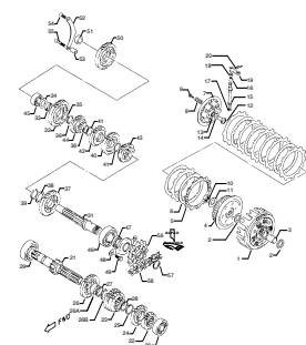
TAV.6 Frizione - Clutch - Embrayage - Kupplung - Embrague
