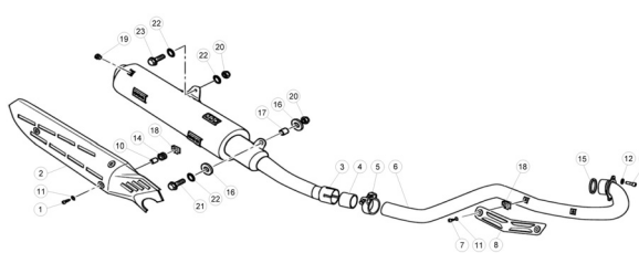
TAV.10 Gruppo scarico - Exhaust system - Echappement - Auspuffanlage - Grupo escape
