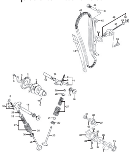
TAV.5 Albero a camme-valvole - Camshaft-Valves - Arbre à cames-Soupapes - Nockenwelle-Ventil - Eje de excentricas-Valvulas
