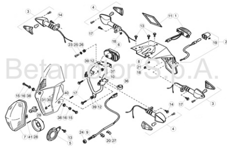
TAV.40B Impianto elettrico - Electrical equipment - Installation électrique - Elektrische anlage - Instalación eléctrica
