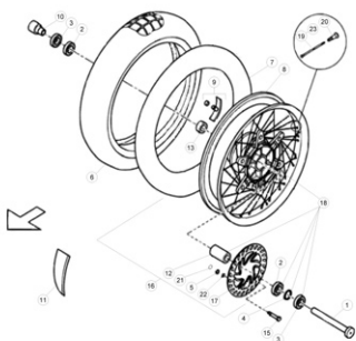
TAV.41 Ruota anteriore - Front wheel - Roue AV. - Vorderrad - Rueda delantera
