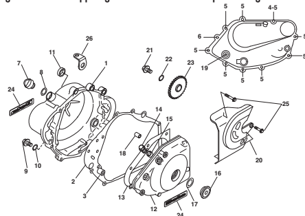
TAV.01A Coperchio frizione-Pignone catena - Clutch cover-Chain sprocket - Couvercle d'embrague-Pignon chaîne - Kupplungsdeckel-Kettenritzel - Tapa embrague-Piñón cadena
