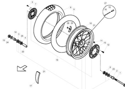
TAV.42 Ruota posteriore - Rear wheel - Roue AR. - Hinterrad - Rueda trasera
