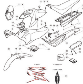
TAV.43 Carenature-Serbatoio-Sella - Fairings-Tank-Saddle - Carenages-Reservoir-Selle - Verkleidungen-Tank-Sattel - Carenados-Deposito-Sillin
