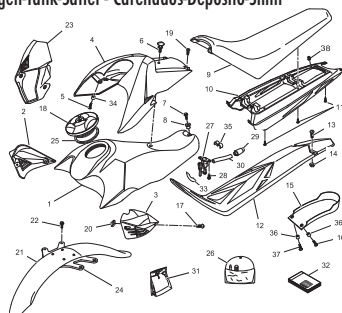
TAV.43 Carenature-Serbatoio-Sella - Fairings-Tank-Saddle - Carenages-Reservoir-Selle - Verkleidungen-Tank-Sattel - Carenados-Deposito-Sillin
