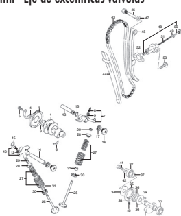
TAV.5 Albero a camme-valvole - Camshaft-Valves - Arbre à cames-Soupapes - Nockenwelle-Ventil - Eje de excentricas-Valvulas
