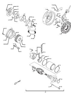
TAV.7 Pompa olio-Volano magnete - Oil pump-Flywheel magneto - Pompe d'huile-Volant magnetique - Olpumpe-Lichtmaschine - Bomba de aceite-Volante magnetico
