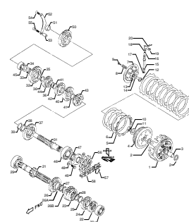
TAV.6 Frizione - Clutch - Embrayage - Kupplung - Embrague
