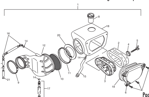
TAV.9 Scatola filtro - Filter box - Boî tier du filtre - Sicherungskasten - Caja del filtro
