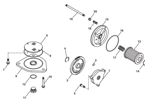
TAV.9 Pompa olio - Oil pump - Pompe d'huile - Ölpumpe - Bomba de aceite
