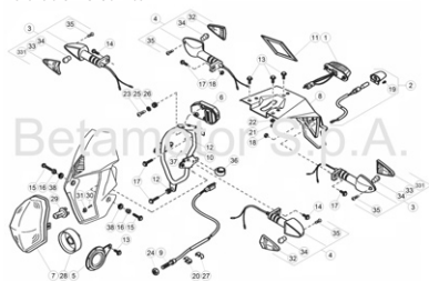
TAV.24 Impianto elettrico - Electrical equipment - Installation électrique - Elektrische anlage - Instalación eléctrica
