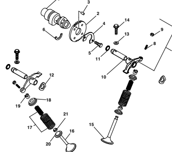
TAV.6 Albero a camme-Valvole - Camshaft - Valves - Arbre à cames-Soupapes - Nockenwelle-Ventil - Eje de eccéntricas-Válvulas
