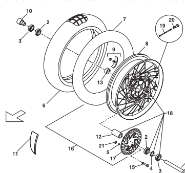
TAV.25 Ruota anteriore - Front wheel - Roue AV. - Vorderrad - Rueda delantera
