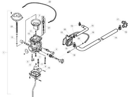
TAV.8A Carburatore - Carburettor - Carburateur - Vergaser - Carburador
