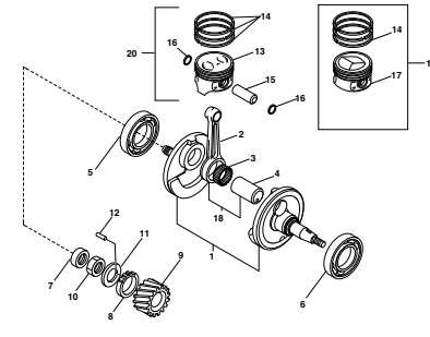
TAV.4 Albero motore-Pistone - Crankshaft-Piston - Vilebrequin-Piston - Kurbelwelle-Kolben - Cigüeñal-Pistón
