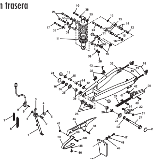
TAV.18 Sospensione posteriore - Rear suspension - Suspension AR. - Hintere aufhängung - Suspensión trasera
