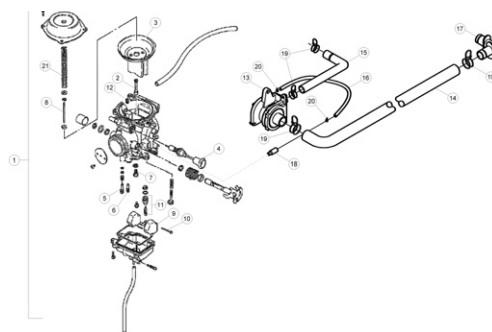
TAV.8 Carburatore - Carburettor - Carburateur - Vergaser - Carburador
