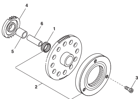
TAV.5 Avviamento - Starter - Dispositif de démarrage - Anlasser - Arranque
