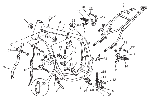
TAV.12 - Telaio-pedane poggiaiedi - Frame-footrests
