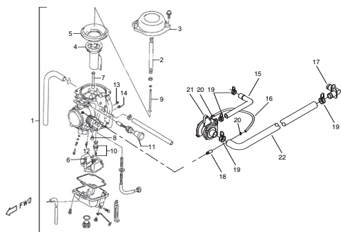
TAV.1 - Carburatore - Carburettor
